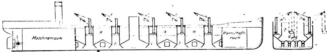
Fig. 6 e 7. - Vapore «Volrath Tham» pel trasporto di mineral.
