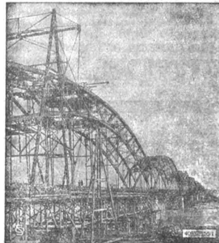
Ponte sul PO alla Geròla (Voghera) lung. m. 751,56. 8 arcate. Fondazioni ad aria compressa.
