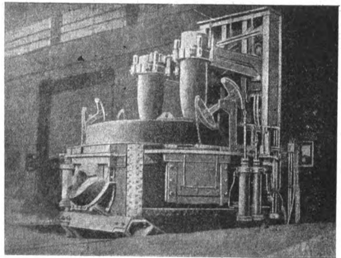
Fig. 3 - Forno da 6 tonnellate.
