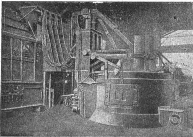
Fig. 2 - Forno trifase da 6 tonn. con regolatore Thury.
