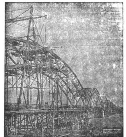
Ponte sul PO alla Gerola (Voghera) lung. m. 751,56. 8 arco. Fondazioni ad aria compressa.
