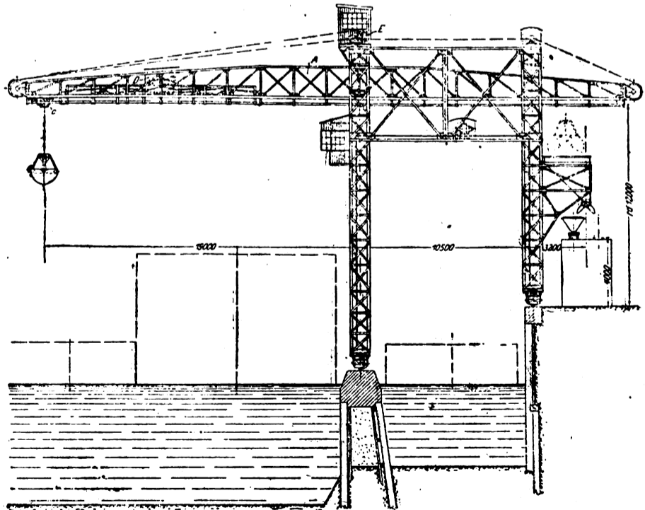
Fig. 1. — Trasbordatore a gru scorrevole in oggetto.
