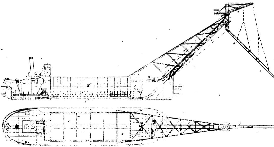
Fig. 19 e 20 - Rifornitore Conrad.
