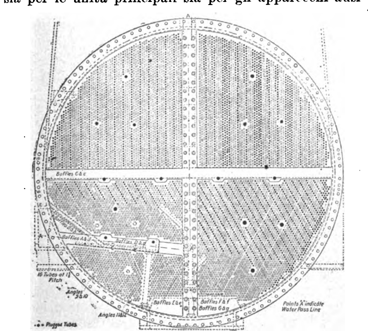
Fig. 16. — Disposizione dei tubi condensatori della Centrale di Connor Creek.
