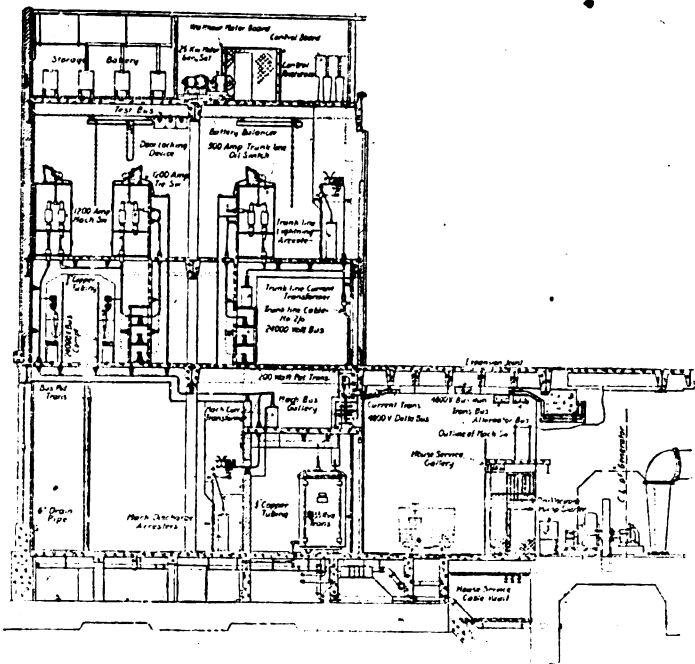
Fig. 18. — Sezione del fabbricato in corrispondenza ai quadri ed ai trasformatori.
