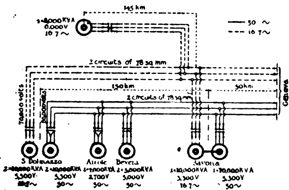
Fig. 4. — Schema del collegamento di due centrali di diverse frequenza della Società Elettrica Riviera di Ponente.
