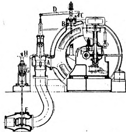
Fig. 2. — Sezione trasversale.
