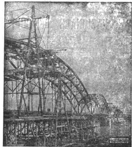
Ponte sul PO alla Gerola (Voghera) ing. m. 751,56. 8 arcate. Fondazioni all'aria compressa.
