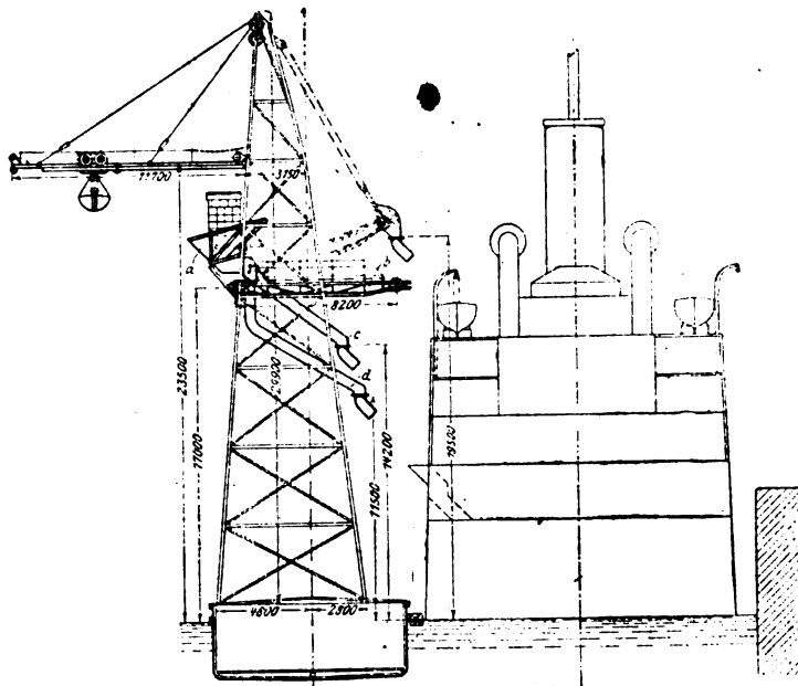
Fig. 29 - Rifornitore con cucchiaino senza elevatore.
