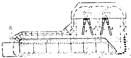
Fig. 14. - Rifornitore e misciatore di carbone galleggiante, tipo Clarke.
