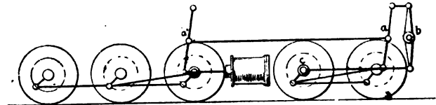
Fig. 8. - Locomotiva a 5 assi Hagans.
