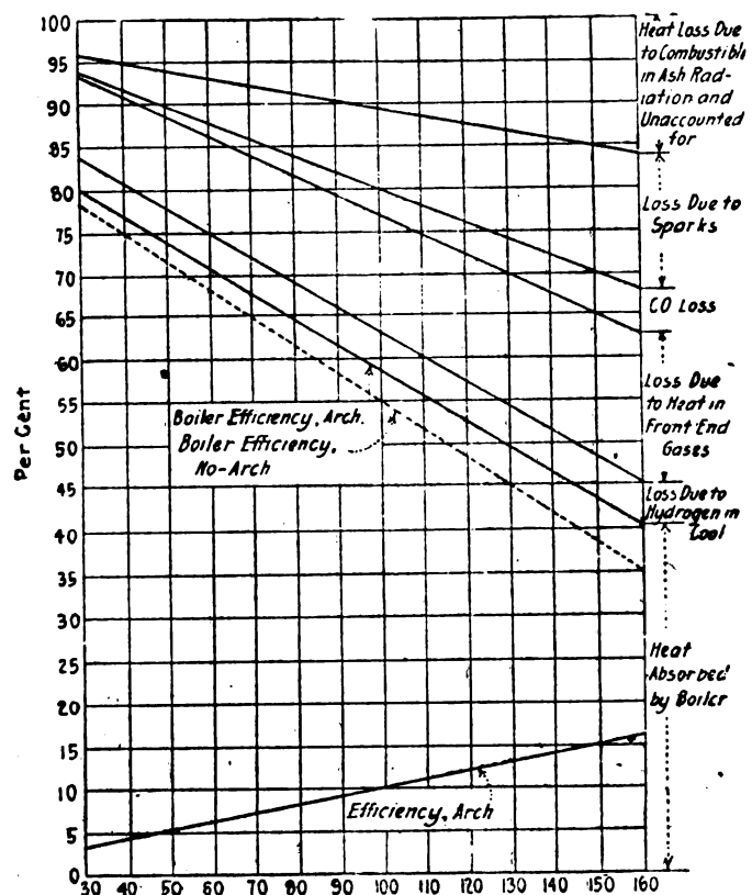
Fig. 2. Rendimento di una caldaia di locomotiva con e senza voltino.
