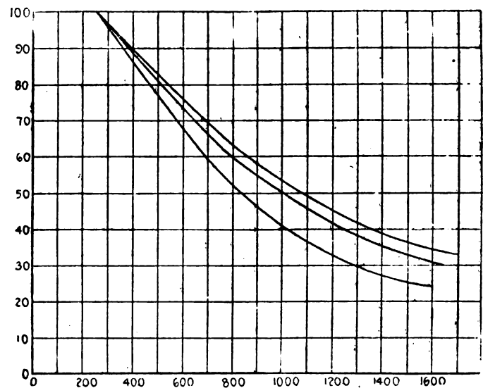
Fig. 1. Rendimento della caldaia con e senza surriscaldamento.
