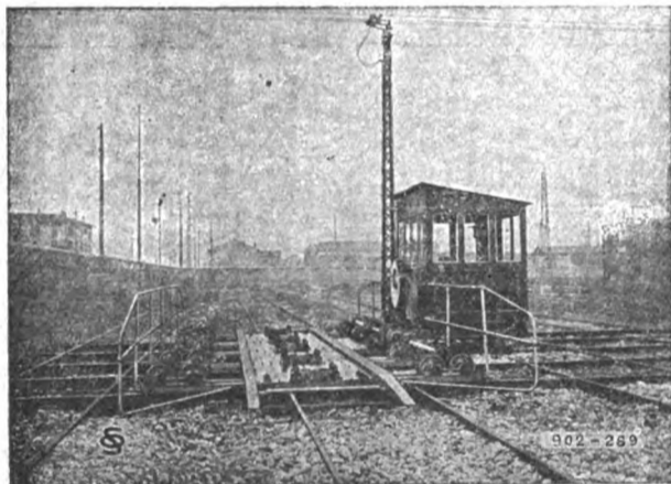
Carrello trasbordatore.
