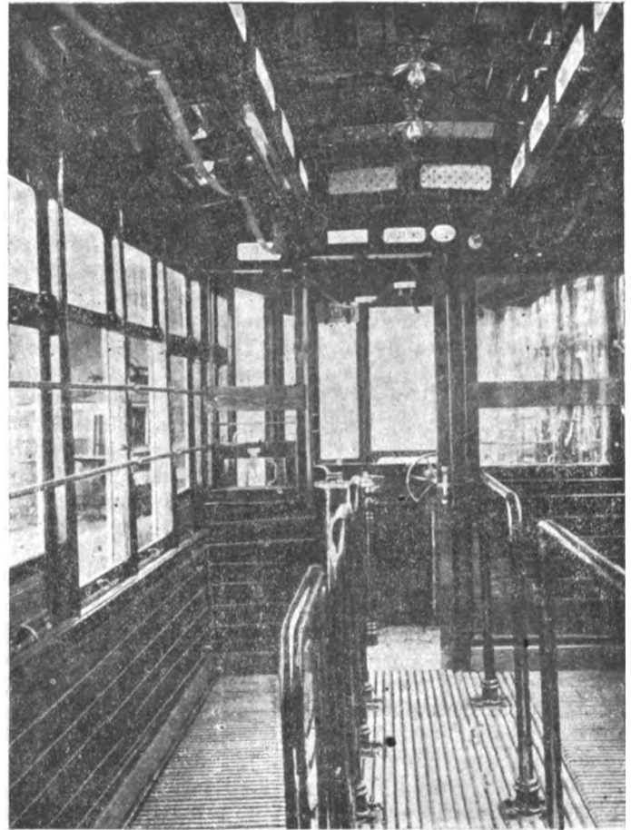
Fig. 1. - Vista dell'interno della vettura trasformata per soli posti in piedi.
