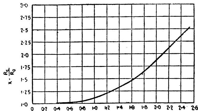
Fig. 1. — Diagramma per la determinazione di x .
