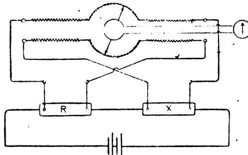
Fig. 3. — Schema dell'apparecchio di Melson per la determinazione della resistenza delle rotaie.
