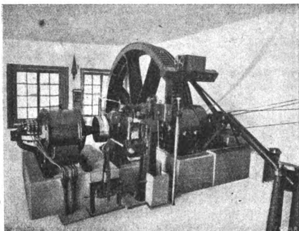
Fig. 3. Macchinario motore.
