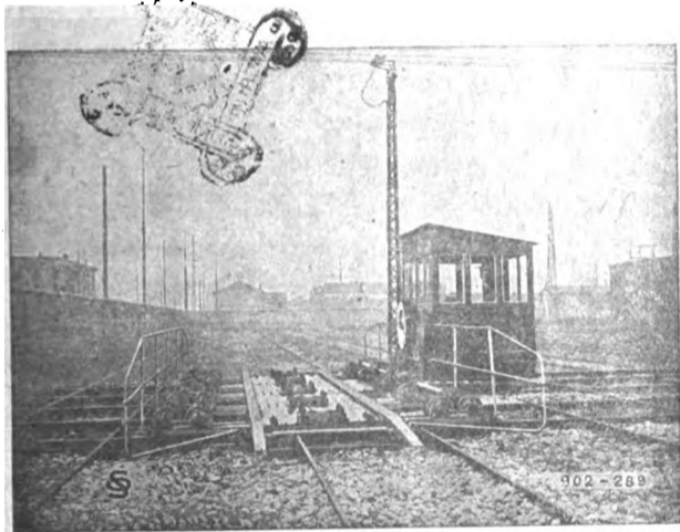
Carrello trasbordatore.
