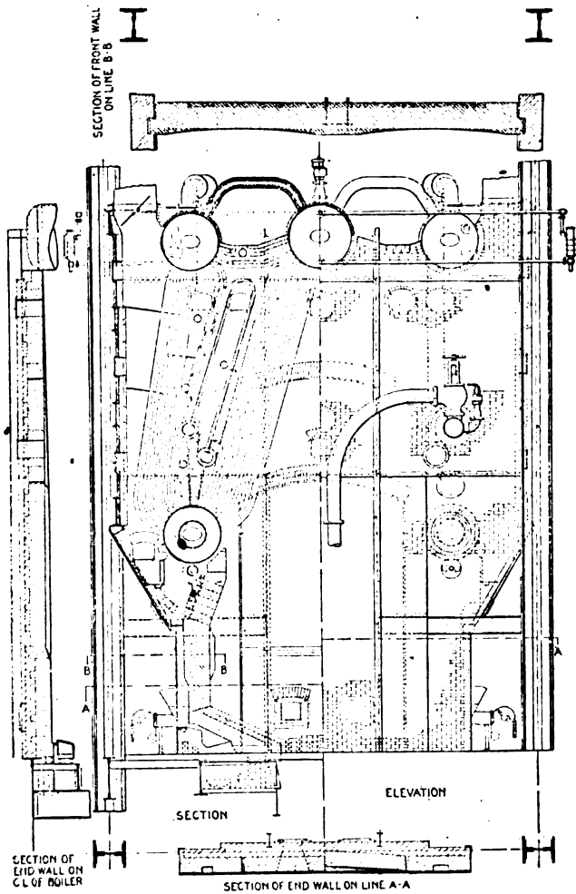
Fig. 15. — Sezioni e vista di una caldaia da 2197 m 2 della centrale di Connor Creek.
