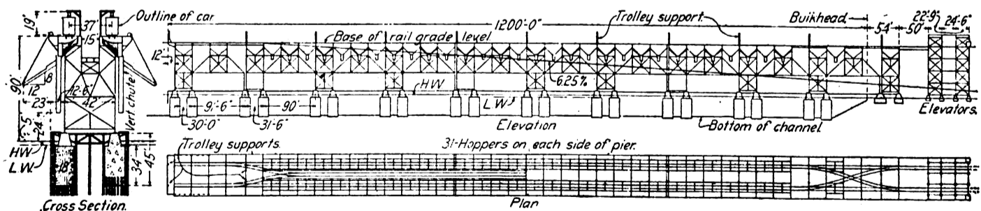
Figg. 80 a 82. - Caricatore di carbone alle navi presso Norfolk.
