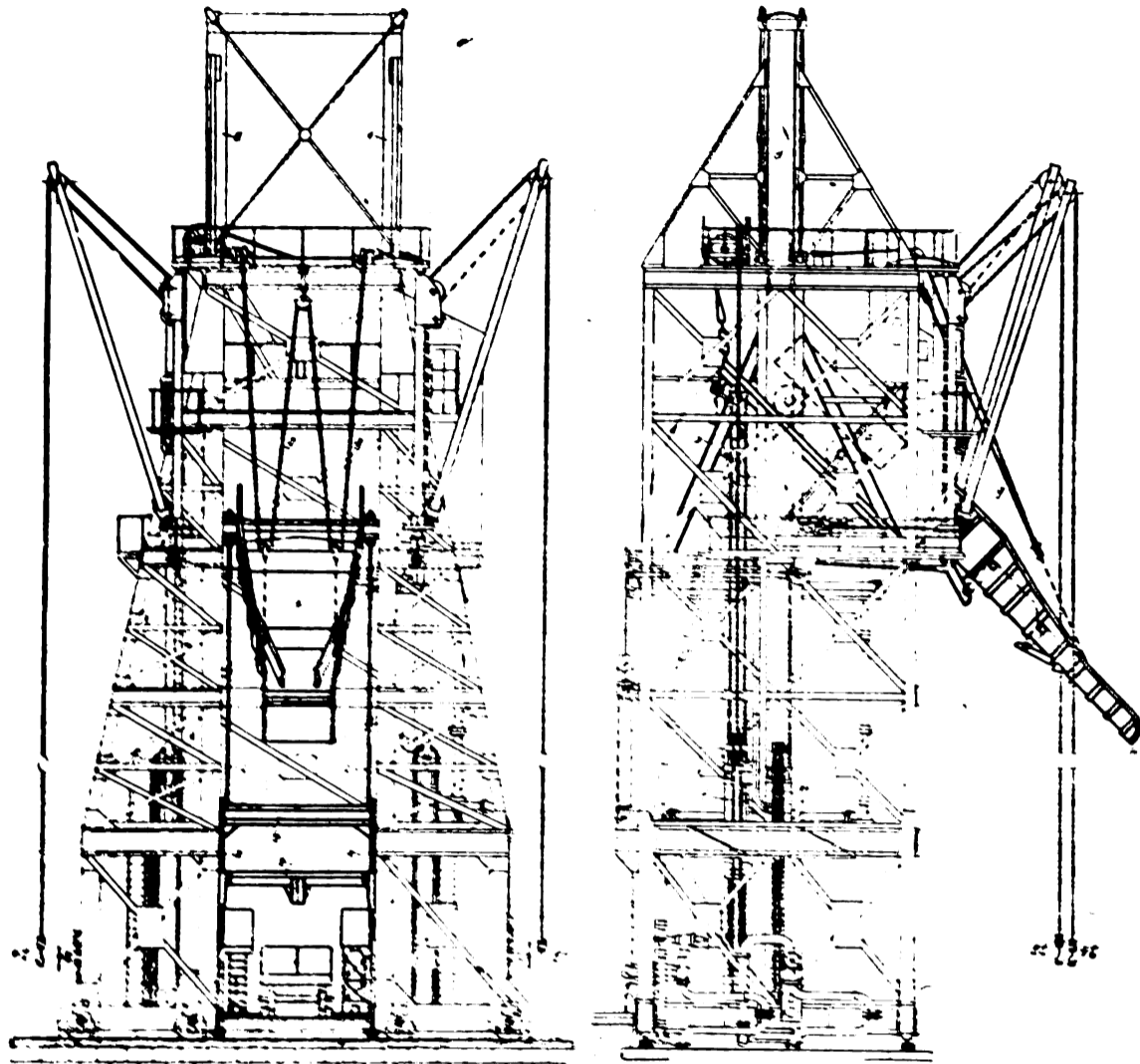
Fig. 1 e 2. — Rovesciatori idraulici scorrenti di Penarth.
