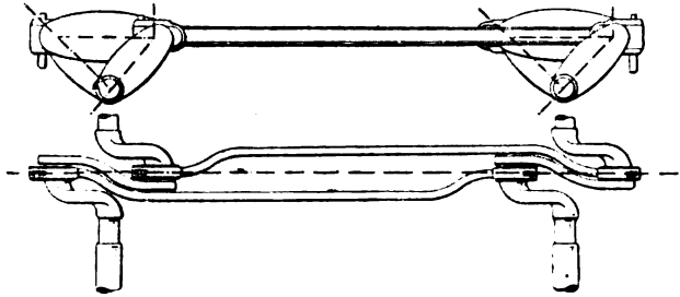
Fig. 6. - Locomotiva Thouvenot.
