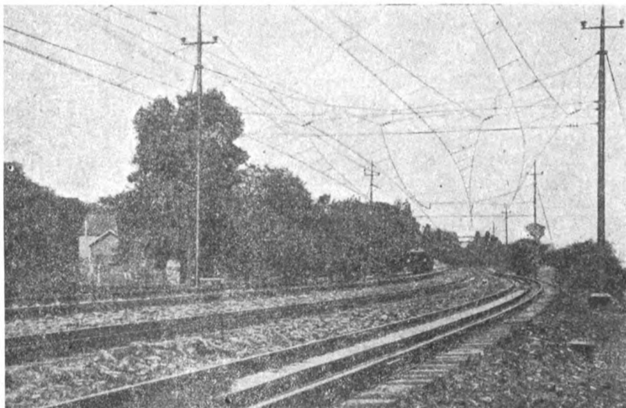
Fig. 8 - Condotte di contatto in curva
