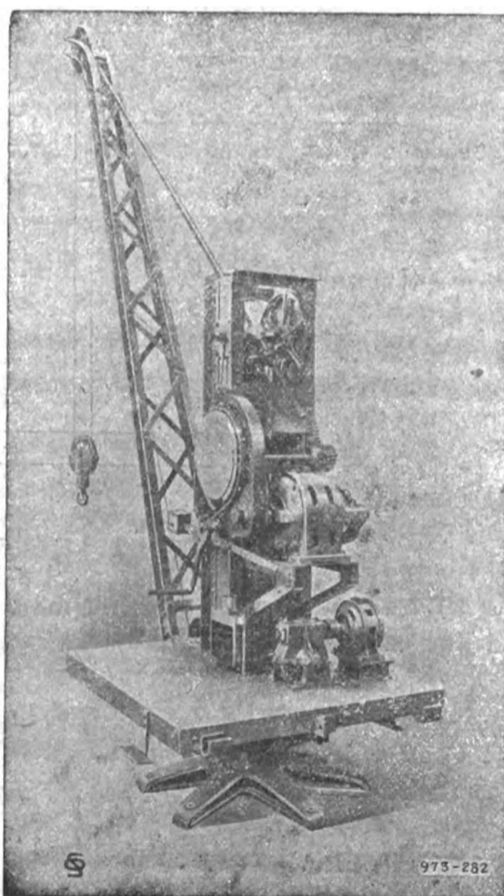
Gru elettrica girevole 3 tonna
