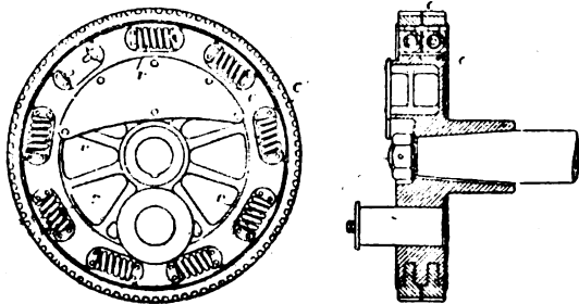
Fig. 2. - Vista e sezione della ruota dentata motrice.
