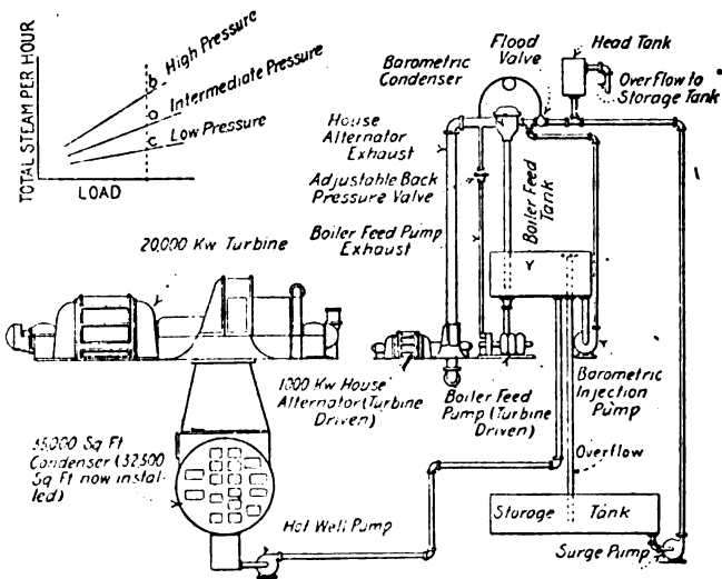
Fig. 17. — Schema della distribuzione dei servizi interni della centrale.
