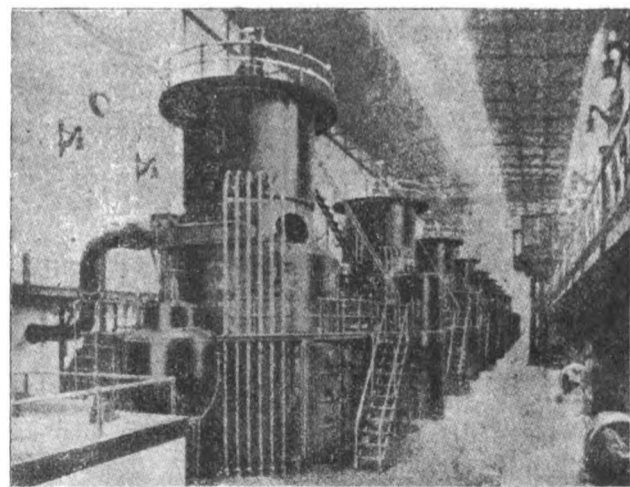
Fig. 7. - Sala delle macchine della Fisk Street Station.
