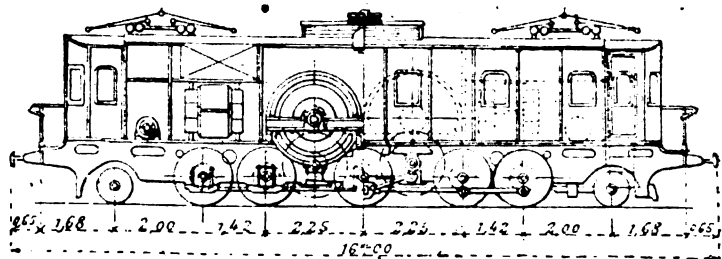
Fig. 3. - Locomotiva di servizio 1 - E - 1 con due motori da 1250 HP.
