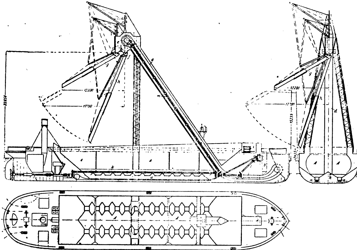
Figg. 21 a 23 - Rifornitore galleggiante con trasportatore a nastri i = bilancia; k, m, l, = alberi motori
