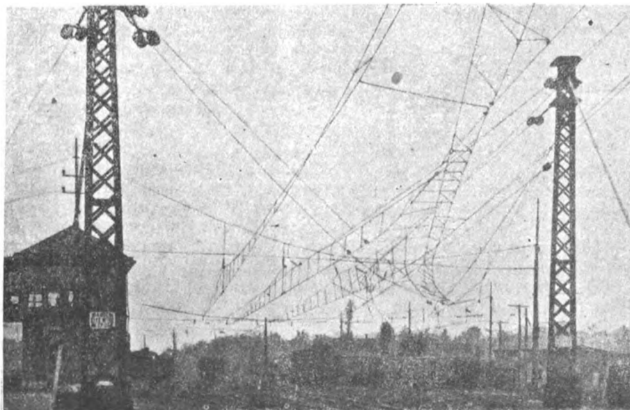
Fig. 9 - Condotte di contatto in un deposito vetture
