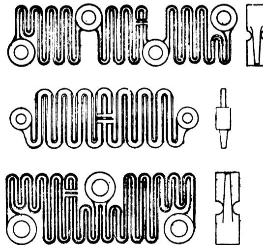
Fig. 1. — Resistenza a griglia di ghisa. (Cy. E. Co).
