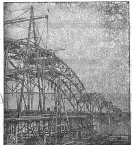
Ponte sul PO alla Gerbia (Voghera) lung. m. 751,56. 8 arcate. Fondazioni ad aria compressa.
