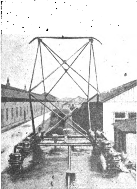
Fig. 15 - Il pantografo
