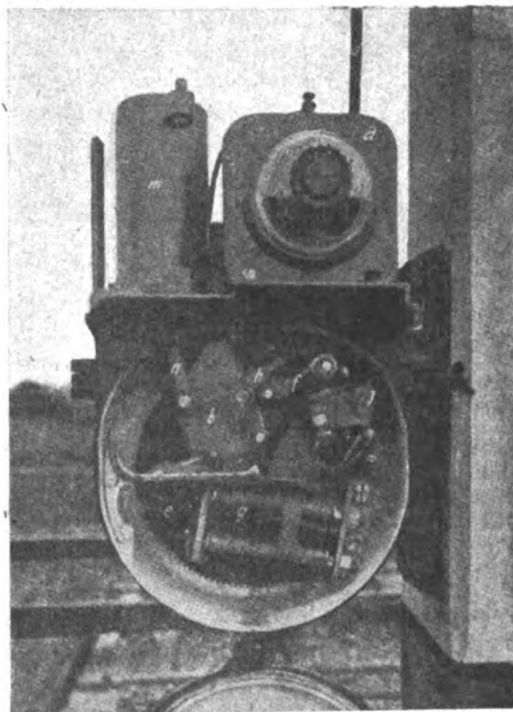
Fig. 4. - Vista anteriore dell'apparecchio di comando del segnale (aperto).
