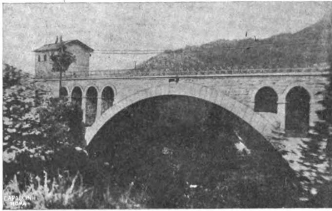
Fig. 7. — Viadotto sulla Valle di Gai, Pr. 41 + 979.
