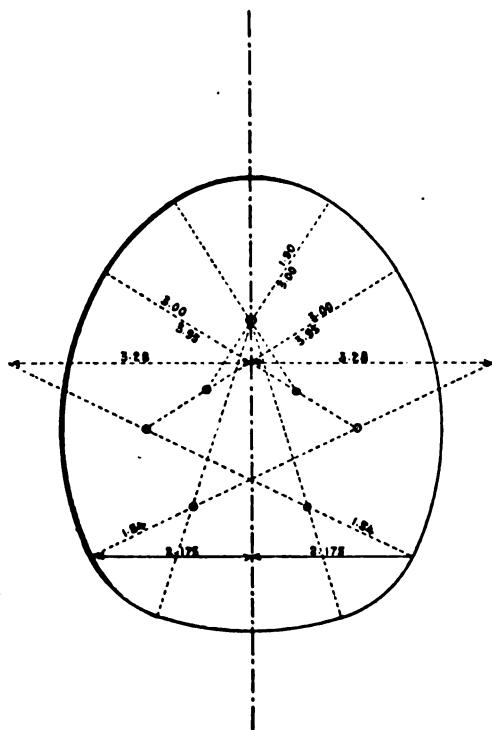
Fig. 20. — Profilo interno della parte mostruata della galleria di Perarolo
