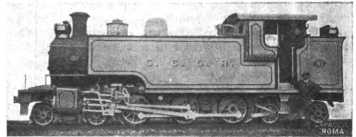
Fig. 19. — Locomotiva tender 4-6-4 per scartamento di 1067 mm. della ferrovia della Costa d'oro.
