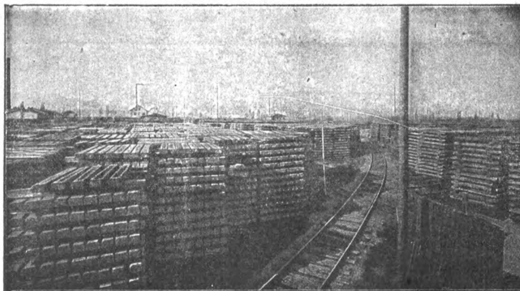
Stabilimento d'iniezione con olio di catrame di Spl-a s. Reno. (Cantiere e deposito delle traverse).
