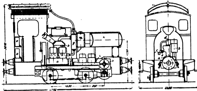
Fig. 25. — Locomotiva Schneider a naftalina.
