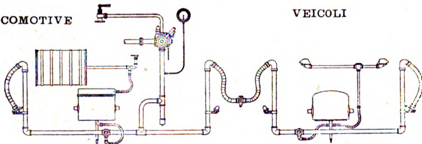
Apparechiatura del freno automatico a vuoto per Ferrovie Secondarie.
