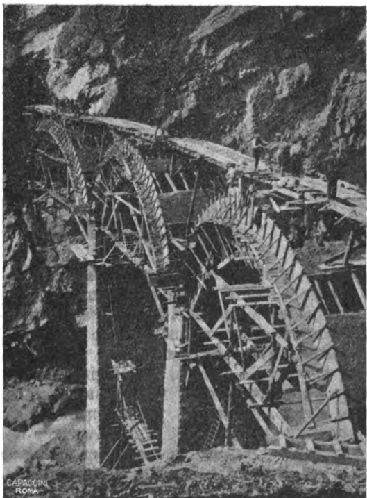
Fig. 3. — Viadotto sul torrente Boite Pr. 36 + 639, durante le gettate dei volti
