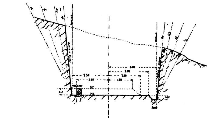
Fig. 3 e 4. - Sezioni normali in trincea in roccia con massicciata incassata.
