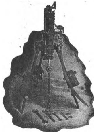
Perforatrice Ingersoll
