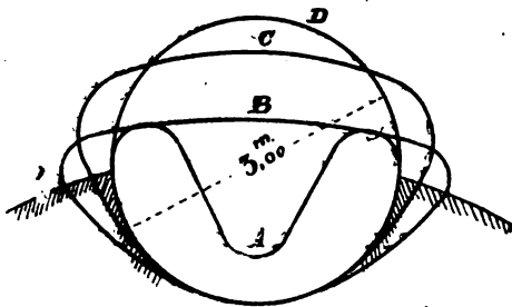
Fig. 3. — Sezioni schematiche della condotta deformata e fasi di ripristino.
