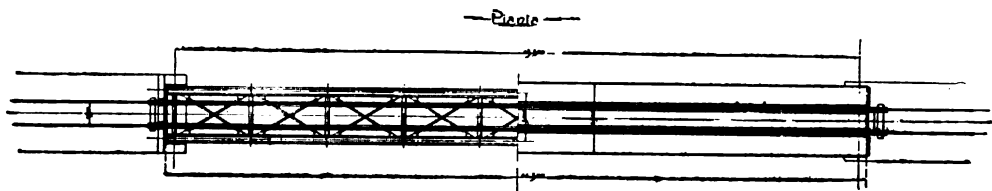
Fig. 5. — Viadotto sulla Busa del Cristo Pr. 88 + 059 - Travate di m. 48,50
