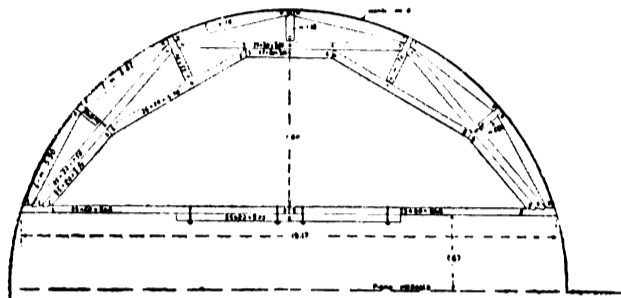
Fig. 9. - Continature per i volti di m. 20,00.
