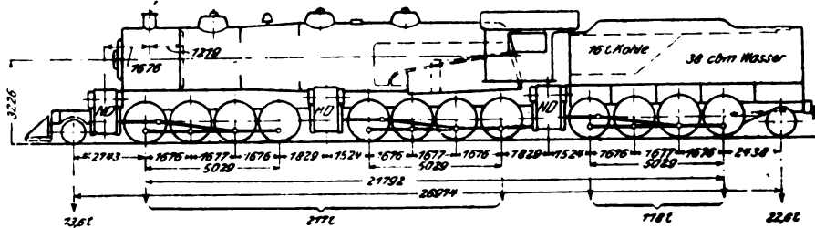
Fig. 18. — Locomotiva Mallet 2-8-8-2 della Ferrovia dell'Erie.
