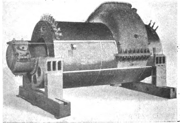
Fig. 4. — Vista esterna della turbina Tosi per Marina.
