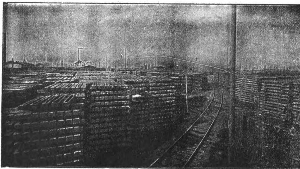
Stabilimento d'iniezione con olio di catrame di Spira s. Reno. (Centriere e deposito delle traverse).
