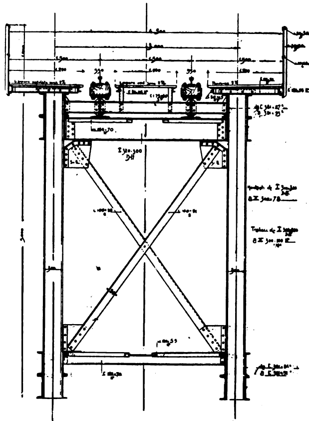
Fig. 6. — Viadotto sulla Busa del Cristo Pr. 88 + 059 Sezione trasversale della travata.
