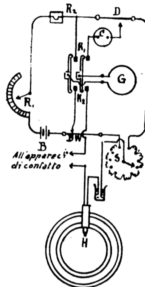
Fig. 8. - Schema delle comunicazioni elettriche per il controllo della temperatura del gas nel cilindro di un motore.
