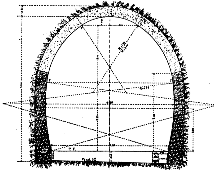
Fig. 12. - Tipo N. 4 - Galleria su terreno ordinario con rivestimento totale.
