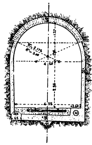
Fig. 11. — Rifacimento di parte della calotta e spadochiature dei piedritti.
