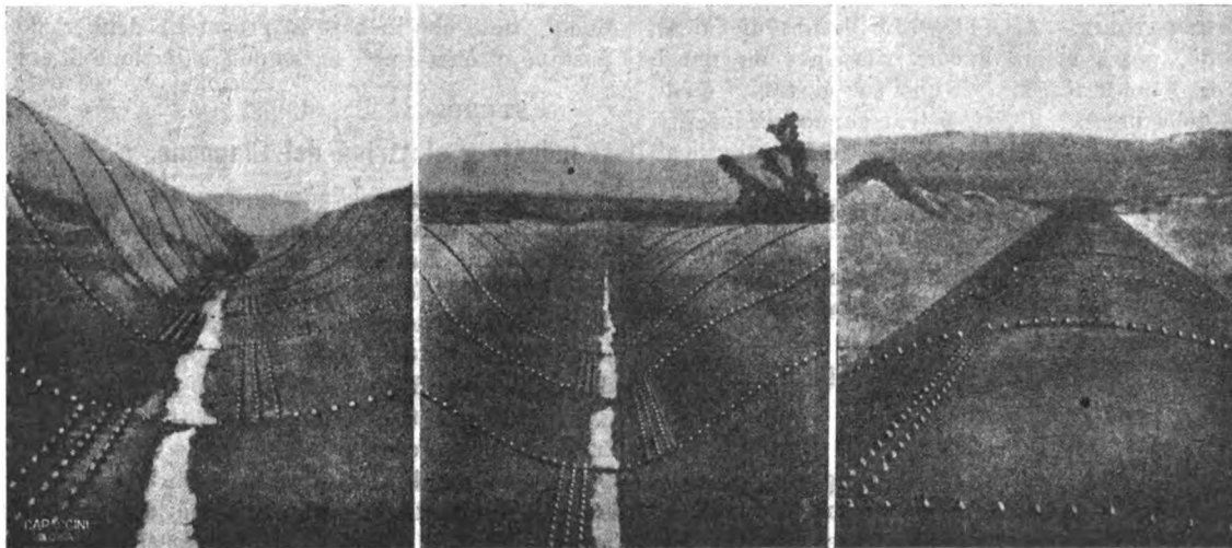
Fig. 4. — Vista della condotta deformata. Fig. 5. — Vista della condotta dopo la prima fase del ripristino. Fig. 6. — Vista della condotta dopo il ripristino.
