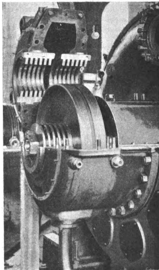
Fig. 11 - Sopperto di spinta aperto.
