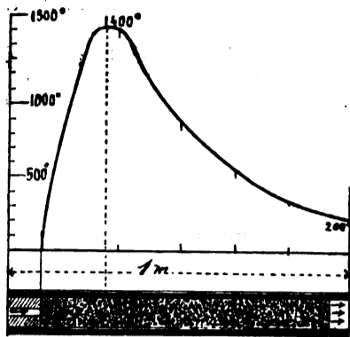
Fig. 1. — Diagramma termico della unità fondamentale.
