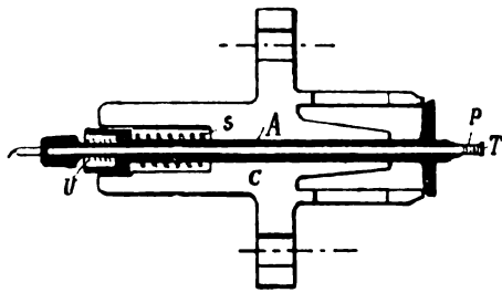
Fig. 1. — Inserzione del termometro nella valvola di ammissione.
