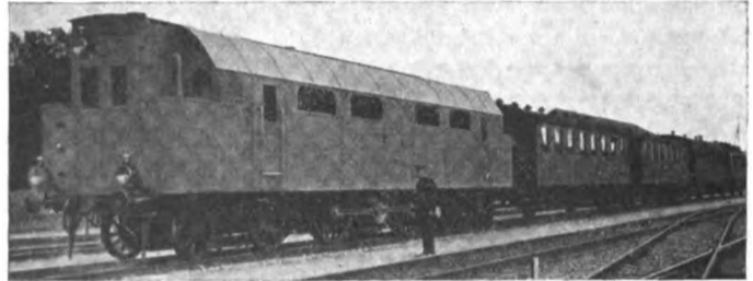
Fig. 7. — Treno di prova sul percorso Winterthur-Romanshorn.
