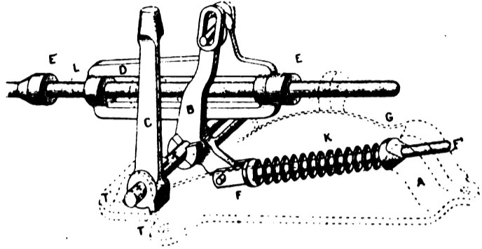
Fig. 10. - Meccanismo di comando dello scambio Beaudenon.
