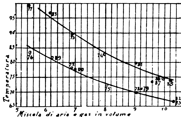
Fig. 7. — Diagrammi delle temperature calcolate lungo la curva di espansione nelle prove a 106 e 200 giri di un motore a scoppio.
