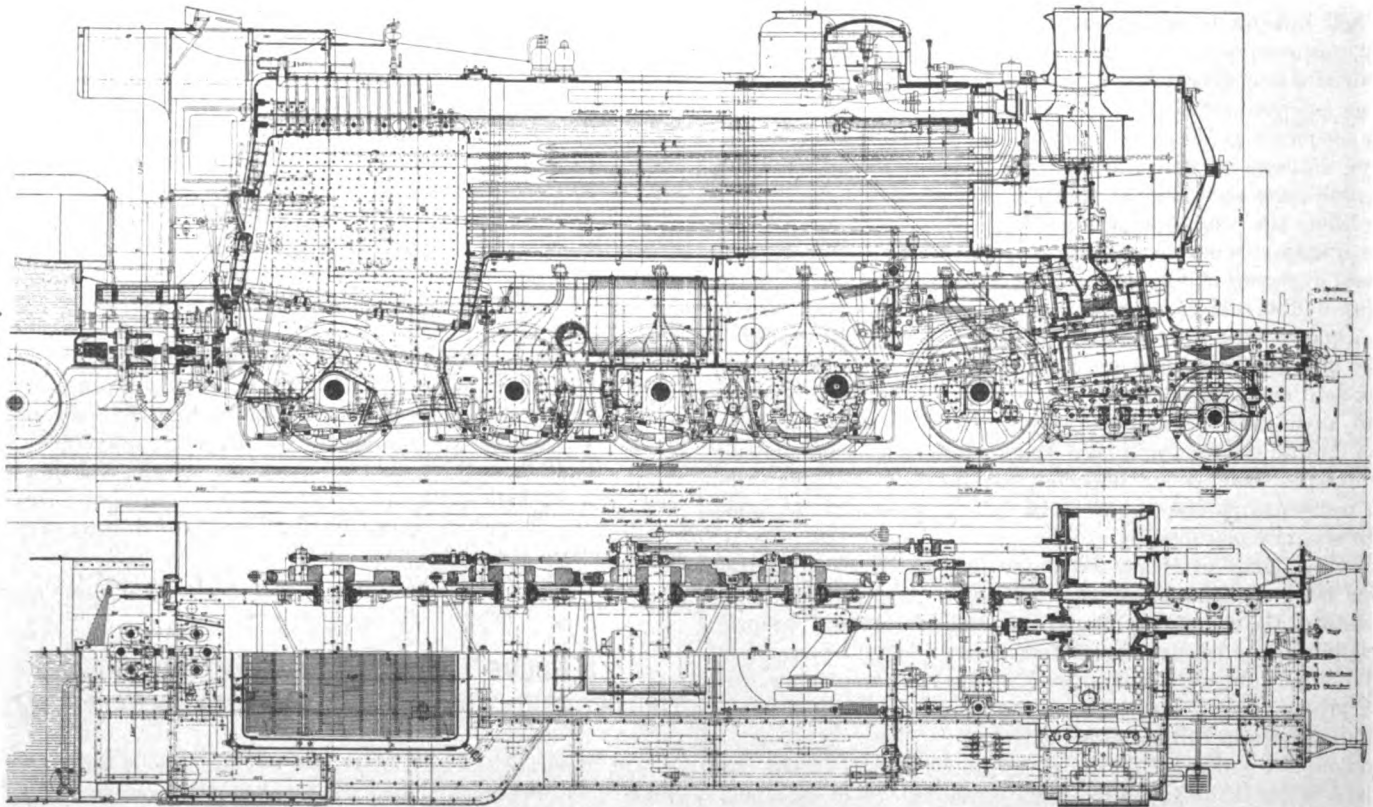
Fig. 11. — Dispositivi della locomotiva decapod serie C 5/6 delle Ferrovie Federali Svizzere.
