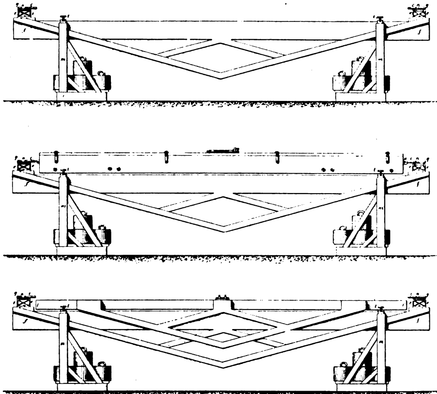
Fig. 14. — Comparatore di Ertel.
