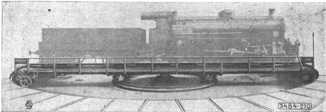
Piattaforma giravole elettrica - Ferrovie dello Stato - Mestre. — Portata 150 tonn. — Diametro metri 21,50.
