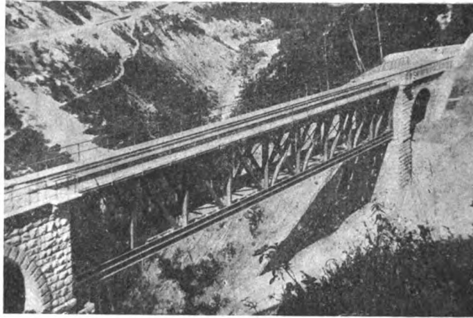
Fig. 4. — Viadotto alla Busa del Cristo Pr. 88 + 059.
