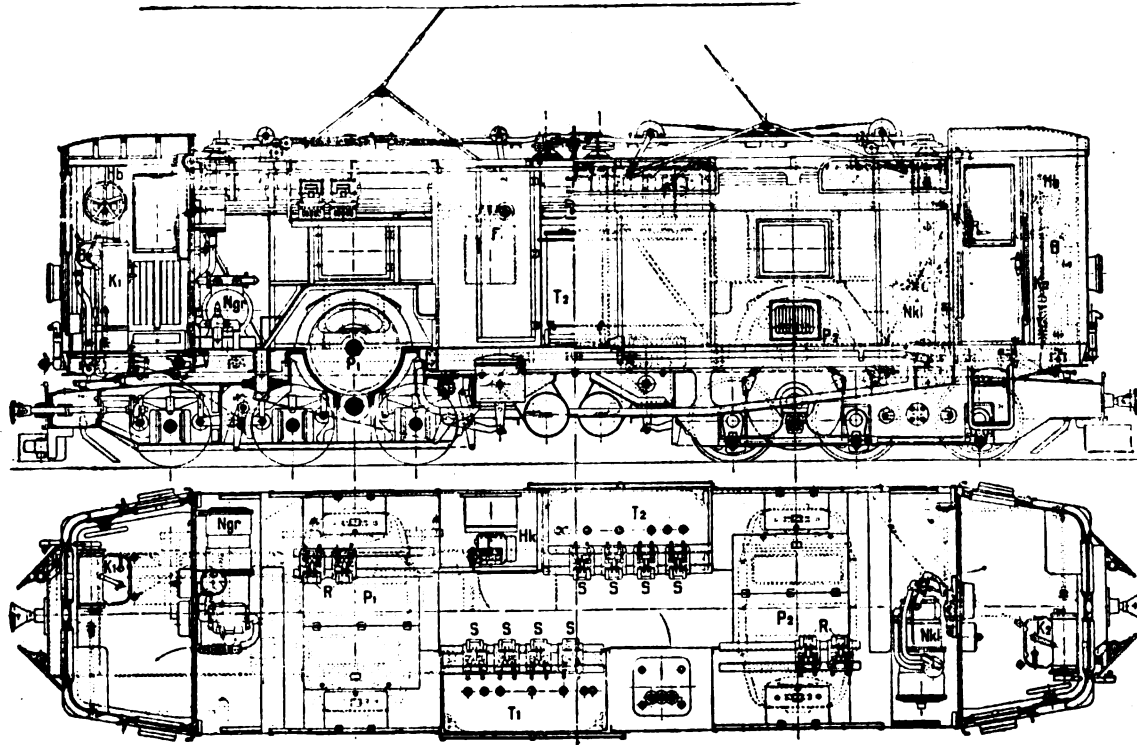
Fig. 5. - Sezione e pianta di una locomotiva.
