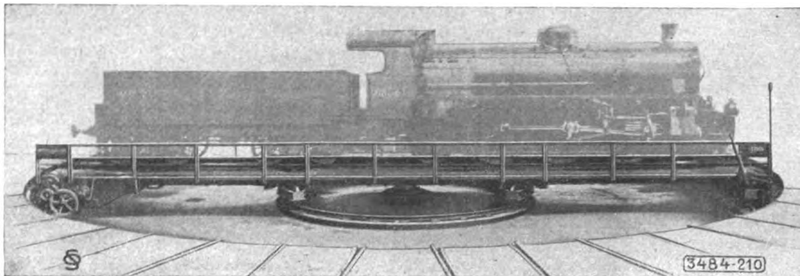
Plattaforma girevole elettrica - Ferrovie dello Stato - Mestre. — Portata 150 tonn. — Diametro metri 21,50.
