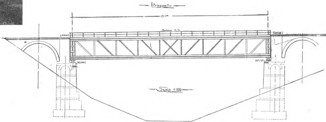
Fig. 2. — Viadotto sul torrente Boite Pr. 36 + 639
