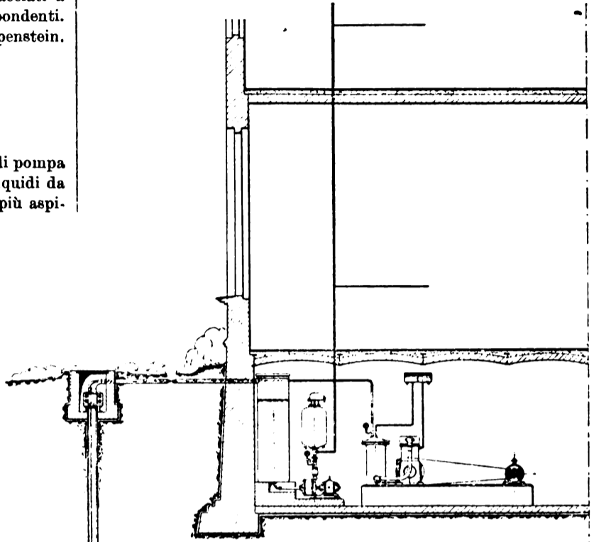
Fig. 12. — Schema dell'impianto di fornitura d'acqua con una pompa Mammut.
