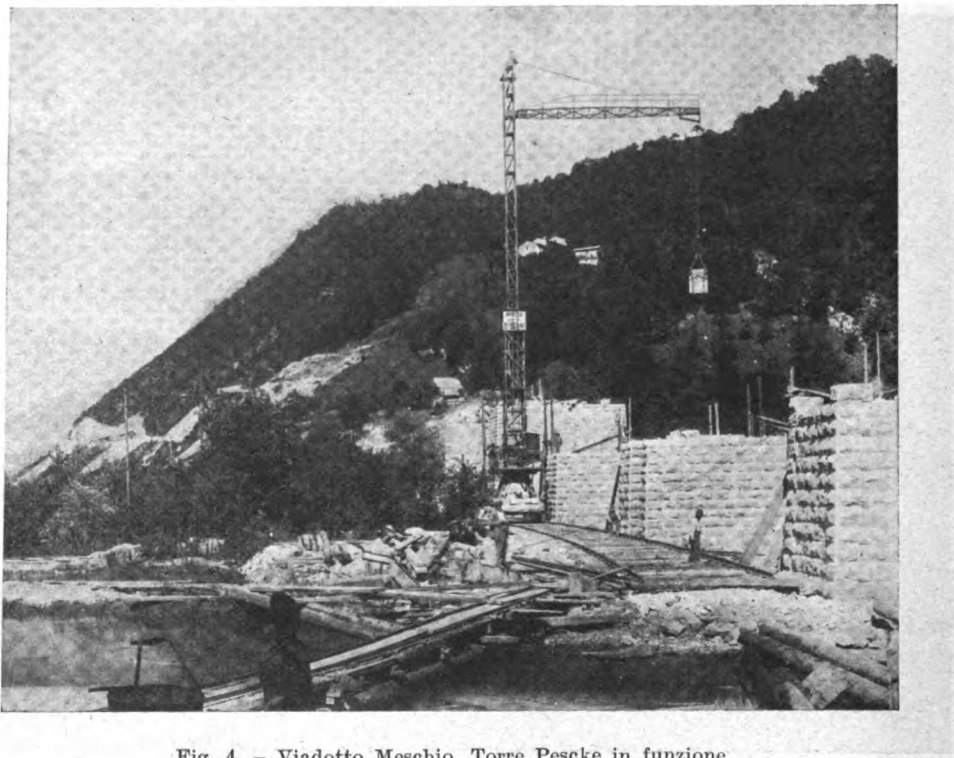
Fig. 4. - Viadotto Meschio. Torre Pescke in funzione.
