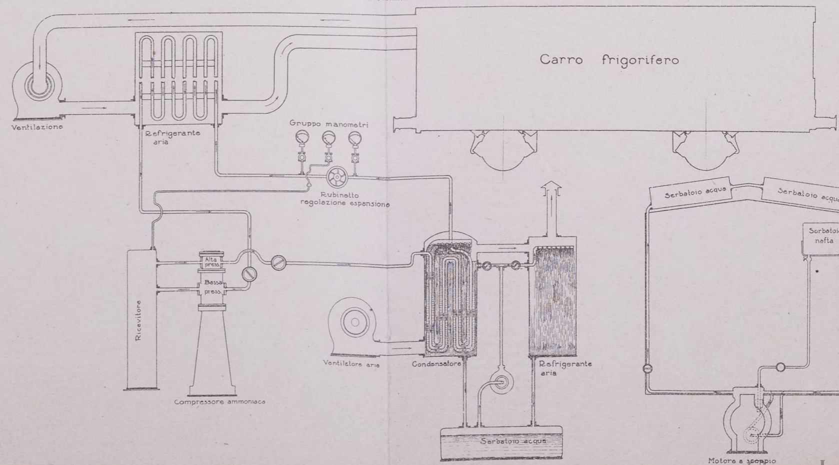
SCHEMA DEI CIRCUITI
