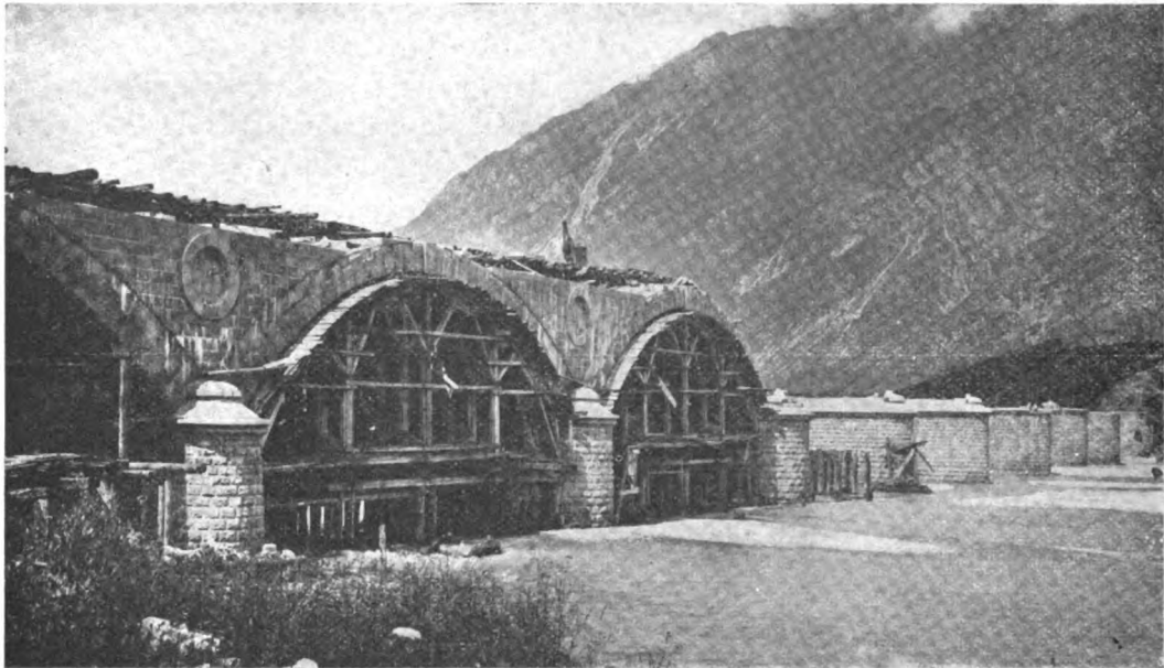
Fig. 6. - Ponte sul Piave. Particolare delle centine.
