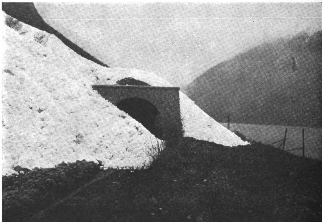
Fig. 11. - Galleria artificiale del Nogher. Imbocco Pont'Alpi, ingombro da una valanga.
