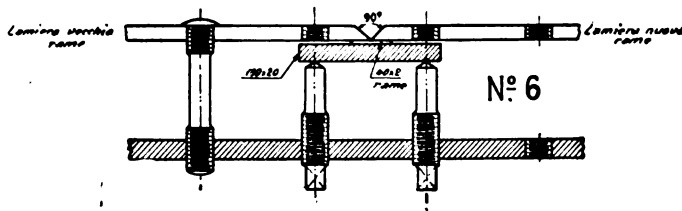
18. Il lamierino di rame e la piastra di ferro devono essere applicati per tutta la lunghezza della saldatura. La piastra di ferro ed i reggicentro filettati vengono smontati ad operazione ultimata.
