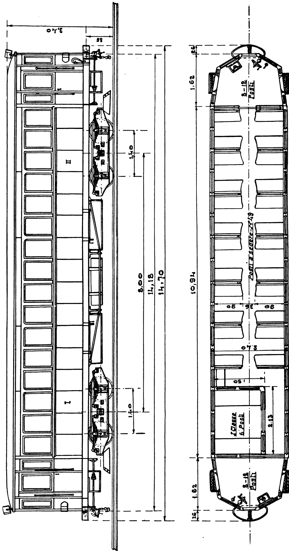
Tramvie provinciali mantovane esercite dall'Amm.ne Prov.le di Mantova. Carrozza automotrice ad accumulatori (4 motori da 30HP ciascuno).
