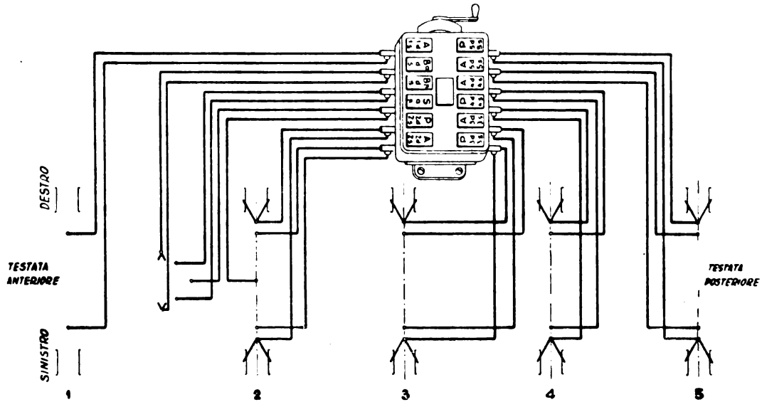
Fig. 1 - Schema delle condotte di lubrificazione delle locomotive Gruppo 713 - 714 delle FF. SS.
