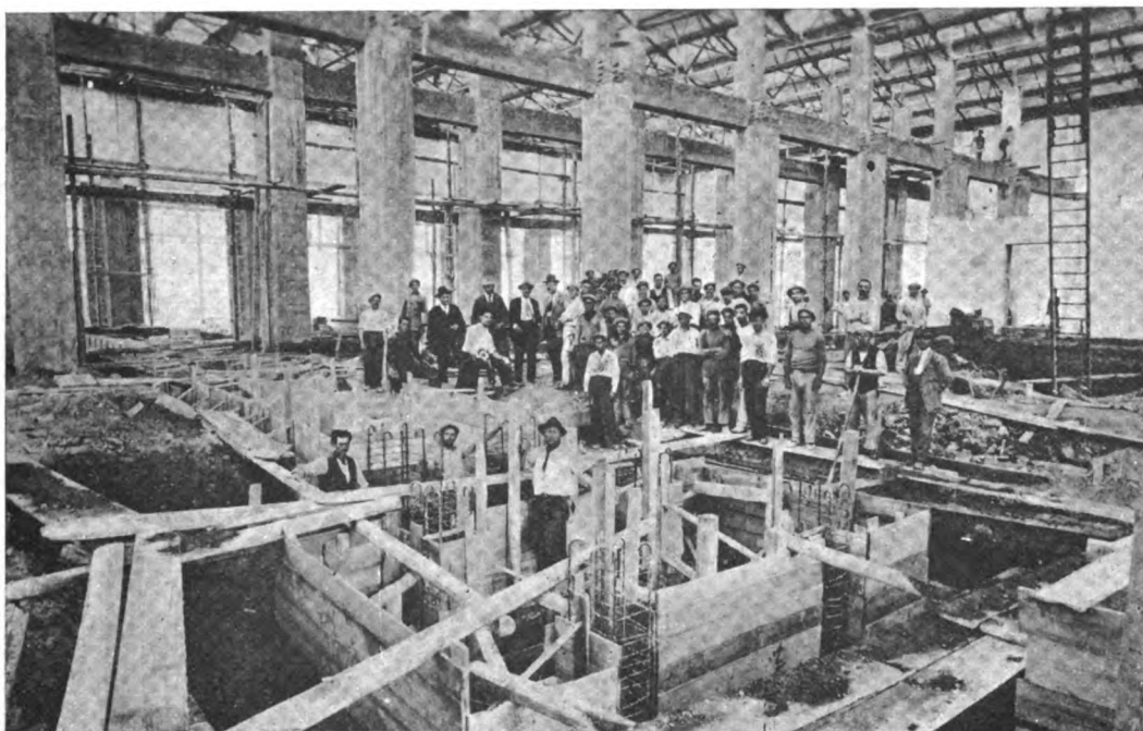
Fig. 7. - Il fabbricato officina e rialzo con una fossa di visita assi durante la costruzione.
