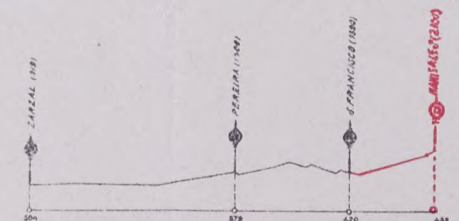
Profilo longitudinale della ferrovia ZARZAL-MANIZALES
