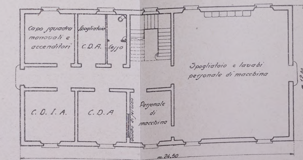
FABBRICATO UFFICI E SCUOLA A. FUOCHISTI
